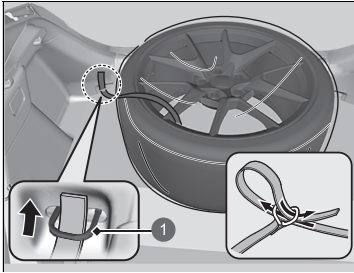
1 Ancre arrière
